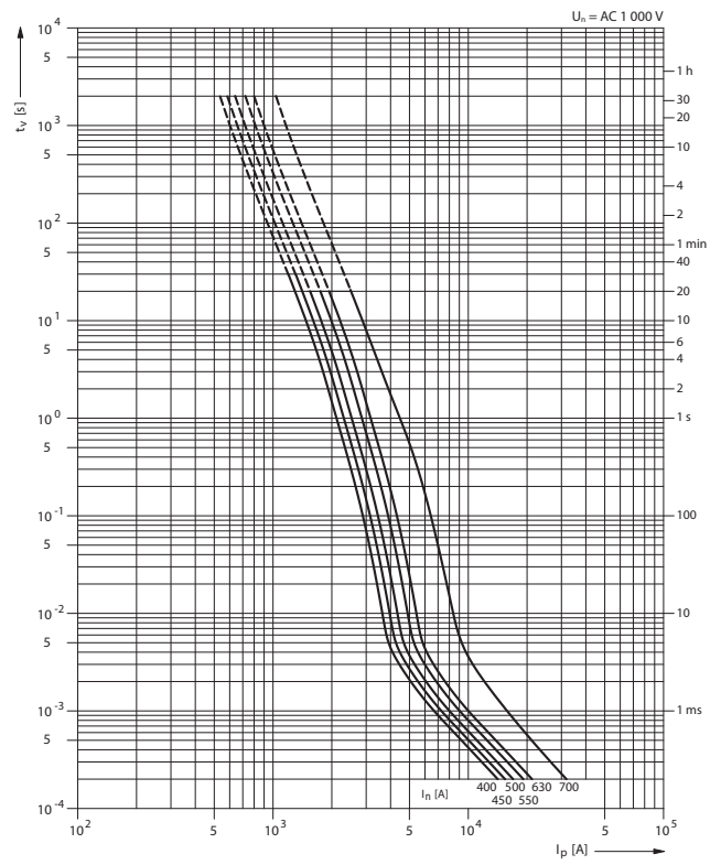
Tavná ampérsekundová charakteristika P50U10, P50V10 aR
