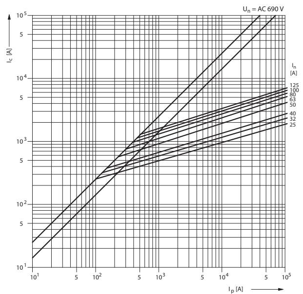
Omezovací charakteristika P50N06 gR, aR
