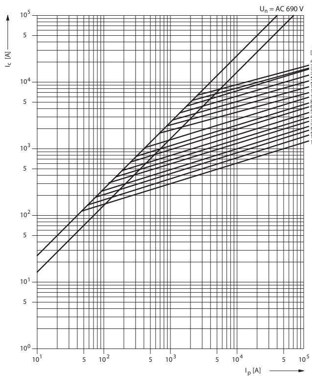
Omezovací charakteristika P50T06 gR, aR
