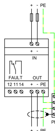
Aplikační schéma zapojení (instalace)
