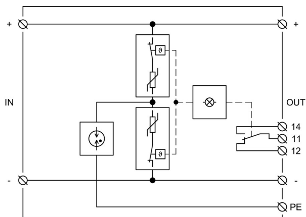
Vnitřní schéma zapojení
