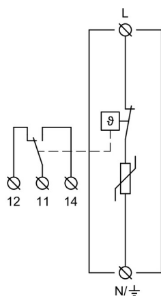
Vnitřní schéma zapojení
