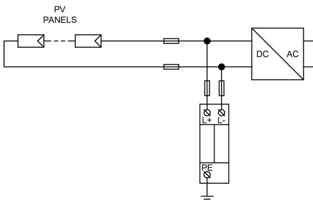
Aplikační schéma zapojení (instalace)
