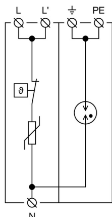
Vnitřní schéma zapojení
