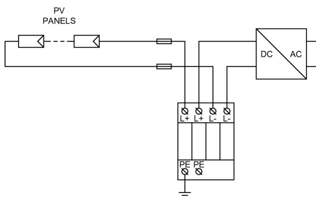
Aplikační schéma zapojení (instalace)
